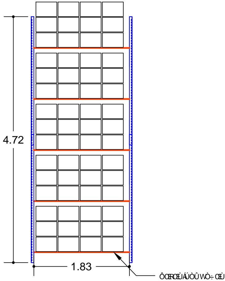
ELEVACION FRONTAL
