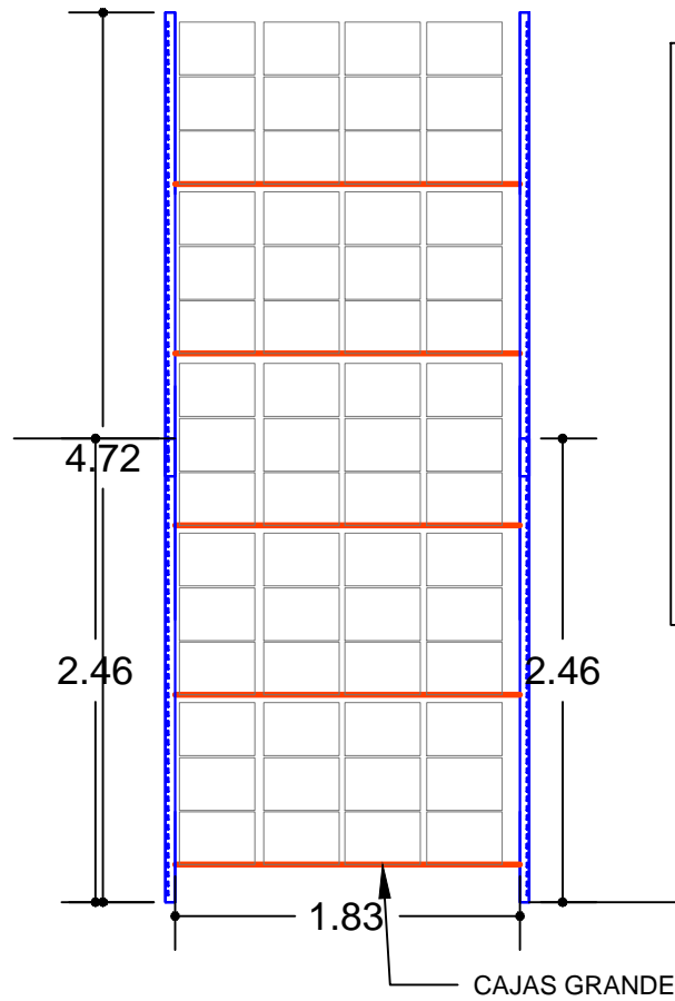
ELEVACION FRONTAL
